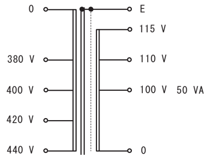
結線図
