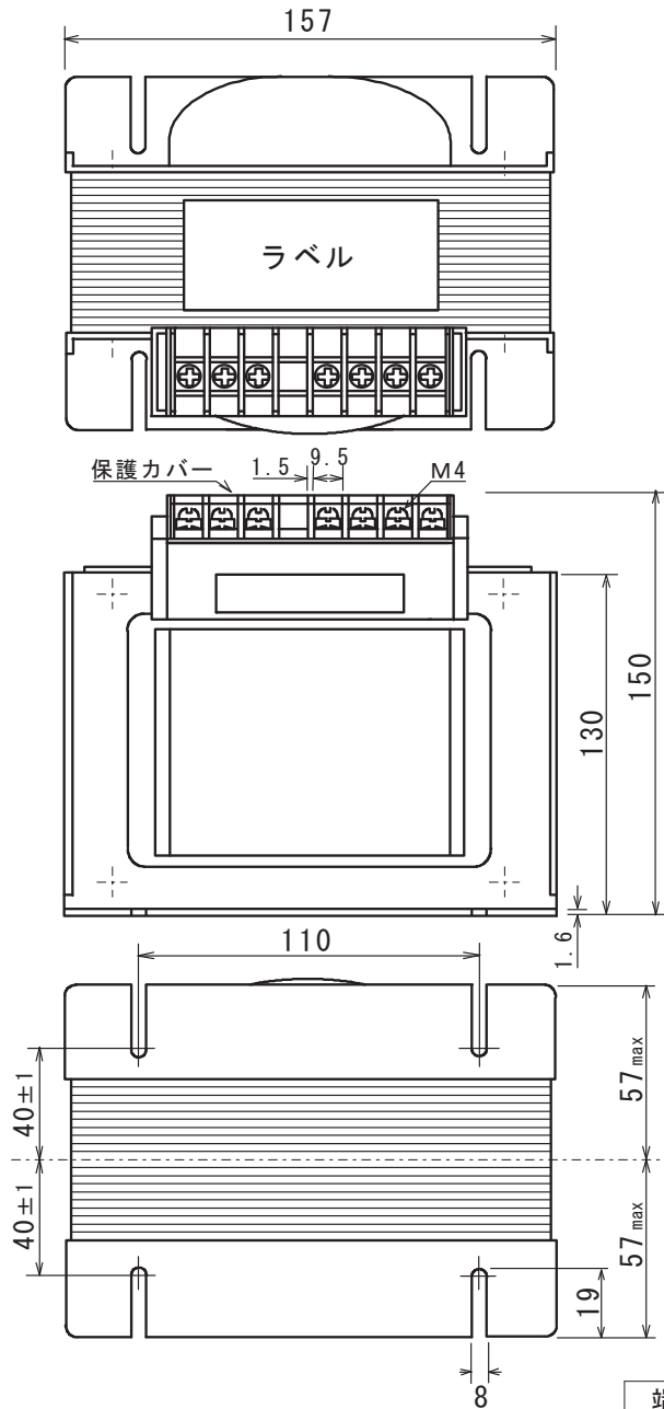
外形寸法図 (単位 mm)
