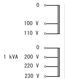
結線図
